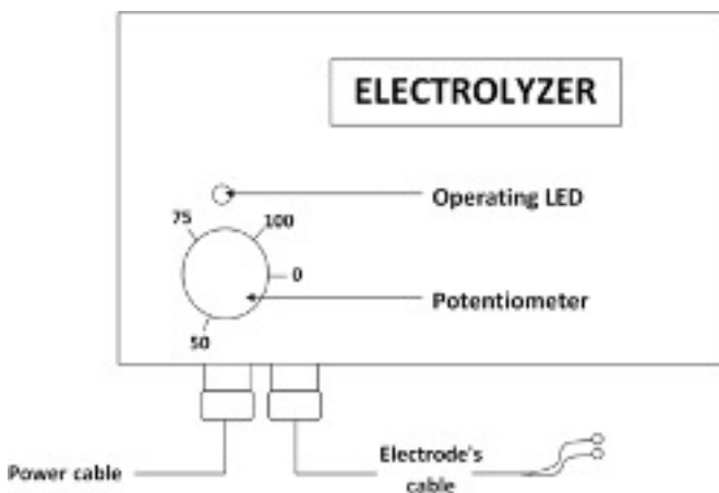
Vorderansicht des Elektrolysegerates
